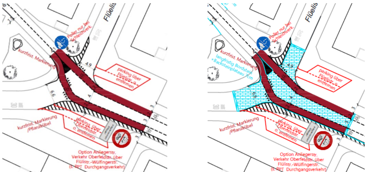
Abbildung 15: VSR 5 Umbau der Knoten Oberfeld-/Wartstrasse, kurz- und langfristig (Team TRIDÉE)
