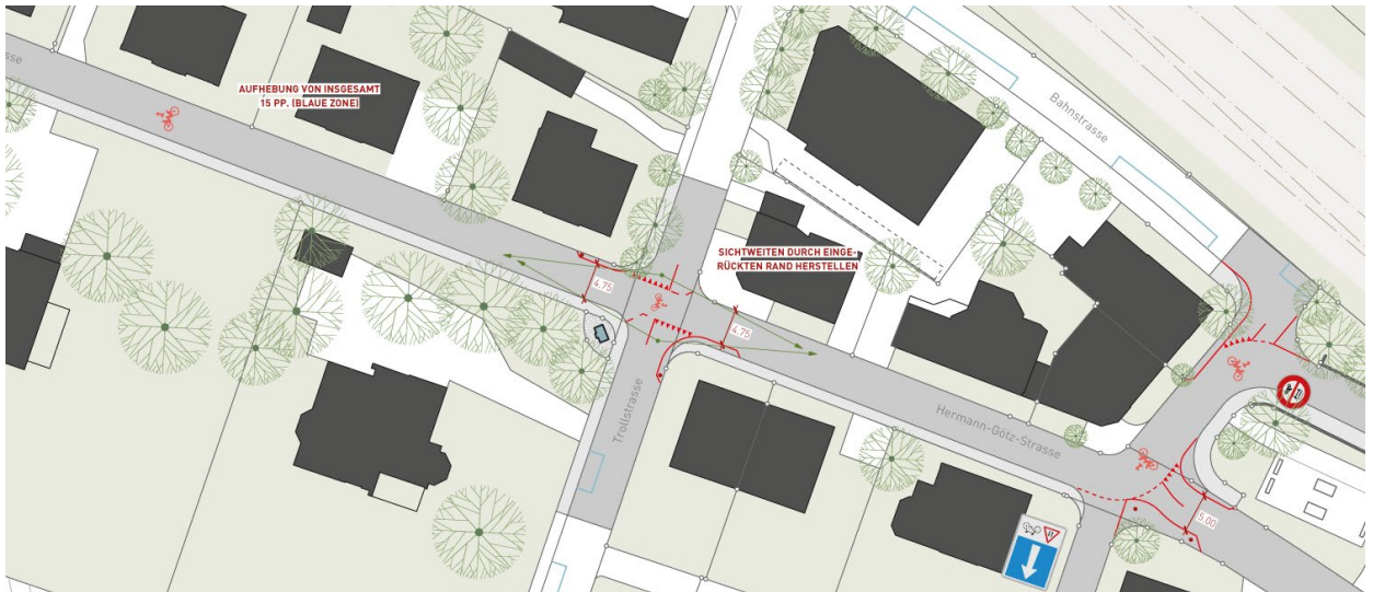
Abbildung 28: VSR 1 Hermann-Götz-Strasse kurzfristig (Team metron)
