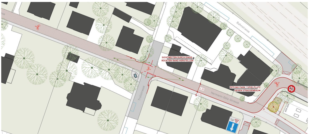
Abbildung 29: VSR 1 Hermann-Götz-Strasse langfristig (Team metron)
