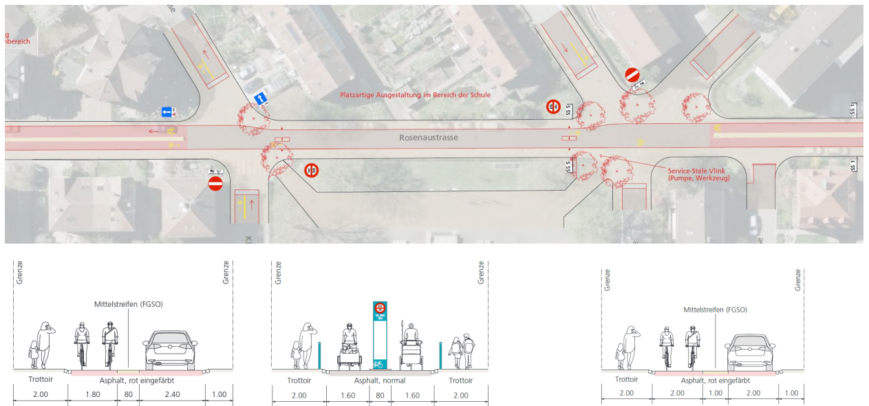
Abbildung 23: Rosenaustrasse Eichliacker, langfristiger Ansatz (asa)
