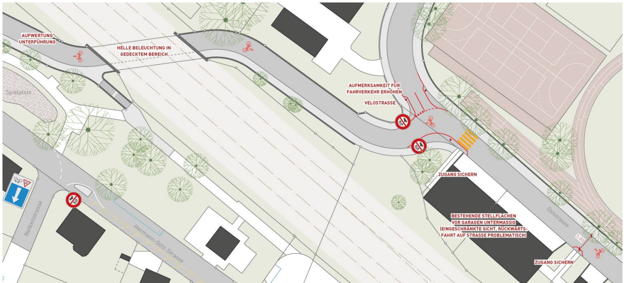
Abbildung 25: VSR 1 Oststrasse, kurzfristig (Team metron)
