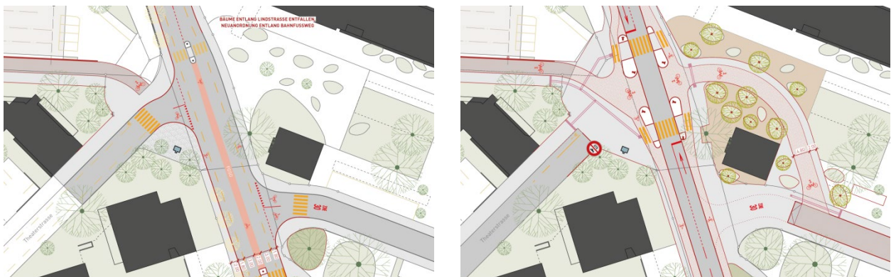
Abbildung 30: Querung Lindstrasse, kurz- und langfristiger Ansatz (Team metron)
