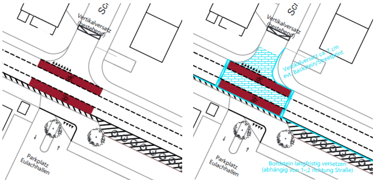
Abbildung 14: VSR 5 Umbau der Knotenpunkte, kurz- und langfristig (Team TRIDÉE)
