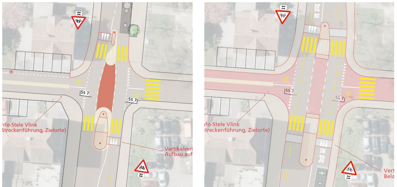
Abbildung 19: VSR 4 Querung Obere Briggerstrasse, kurz- und langfristige Lösung (Team asa)
