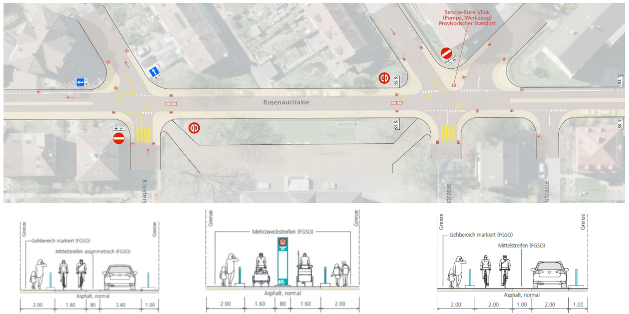
Abbildung 22: Rosenaustrasse Eichliacker, kurzfristiger Ansatz (asa)
