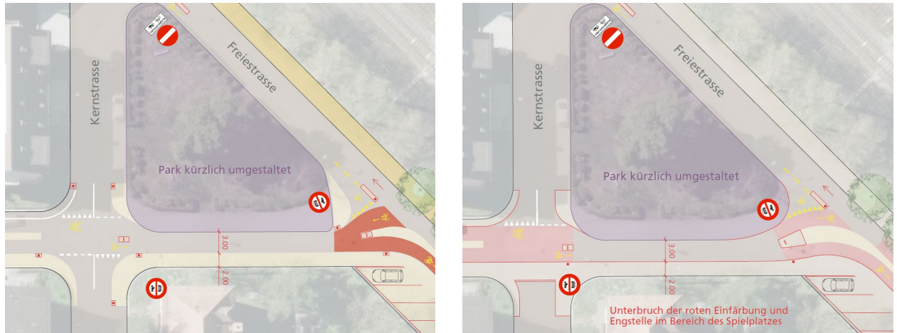
Abbildung 21: Bereich Rosenau-/Kern-/Freiestrasse, kurz- und langfristige Lösung
