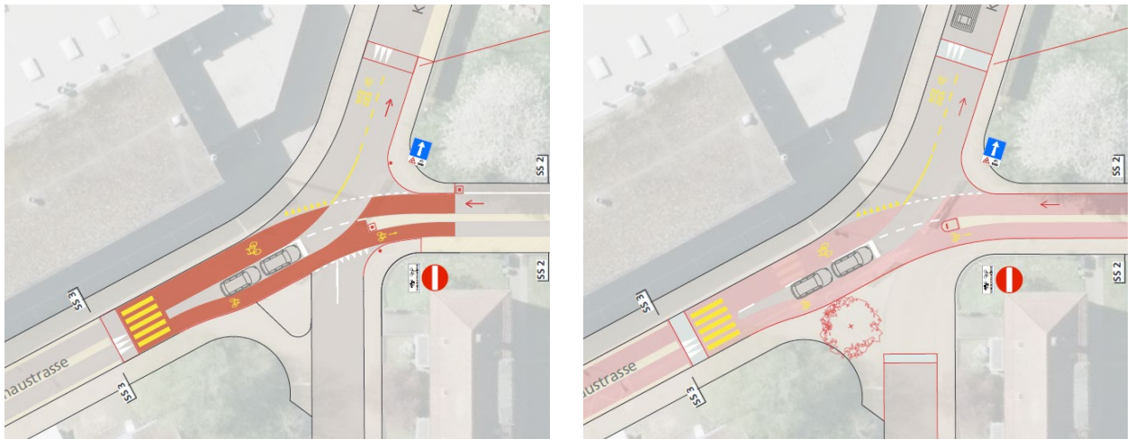
Abbildung 24: Rosenau-/Krummackerstrasse, kurz- und langfristiger Ansatz (Team asa)
